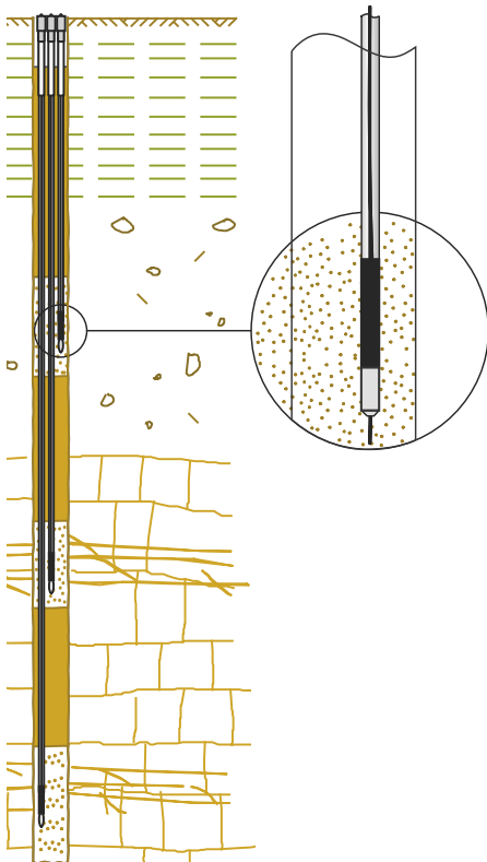
孔隙水压力系统安装示意图
